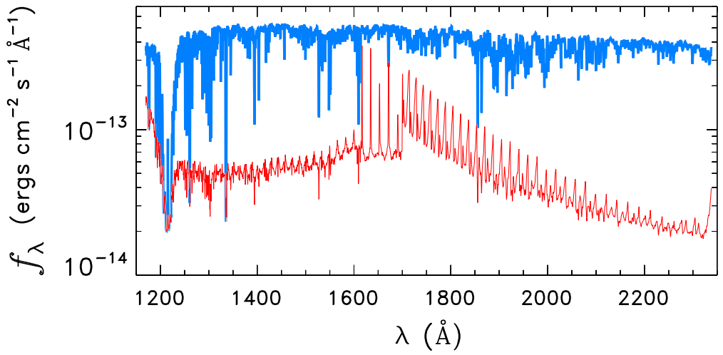
STAR0104-7206
