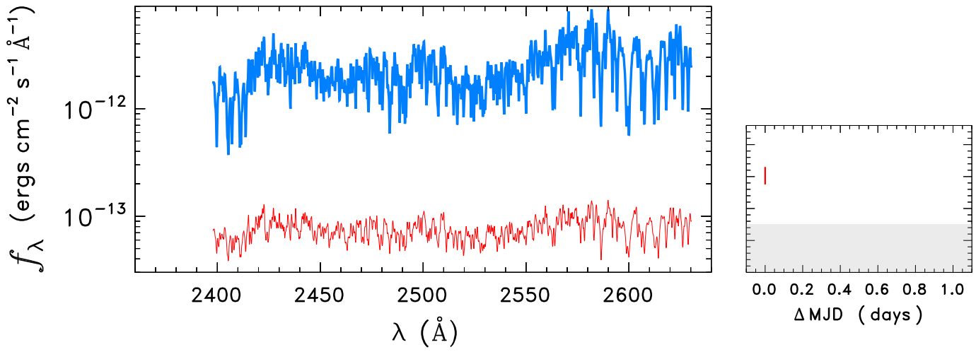
HD198084
