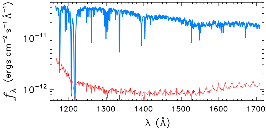
HD146813
