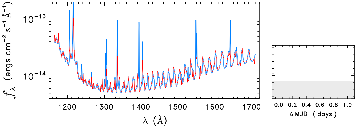
HD43162
