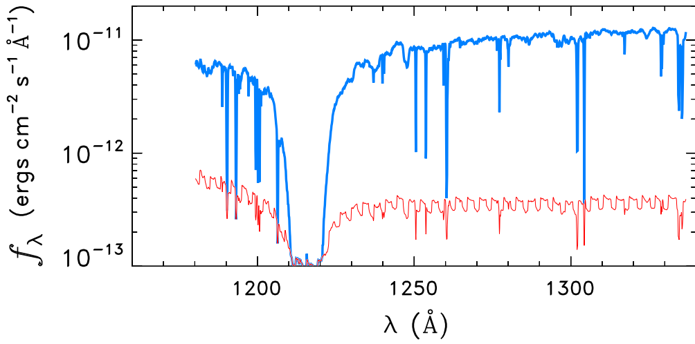
HD115071
