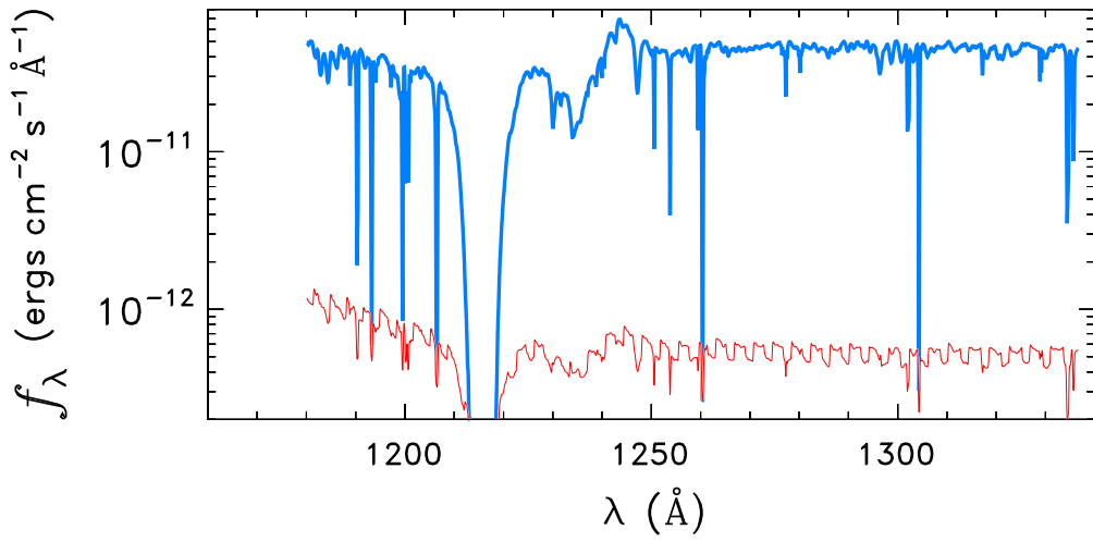
HD116852
