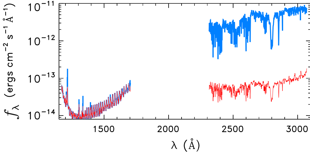
HD106516
