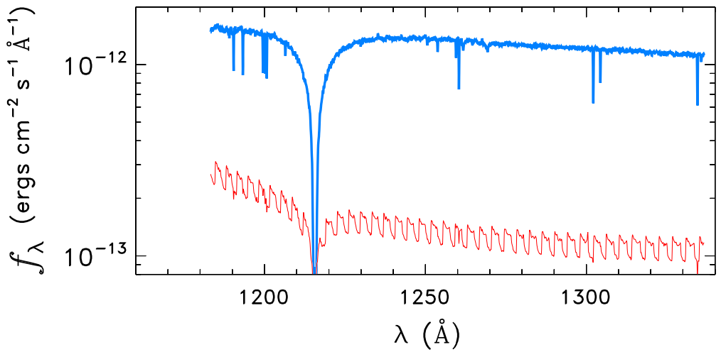
WD1123+189
