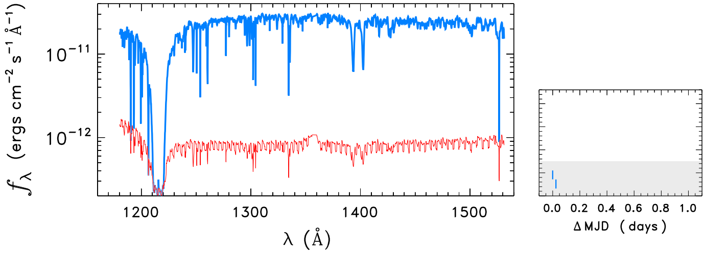
HD108639
