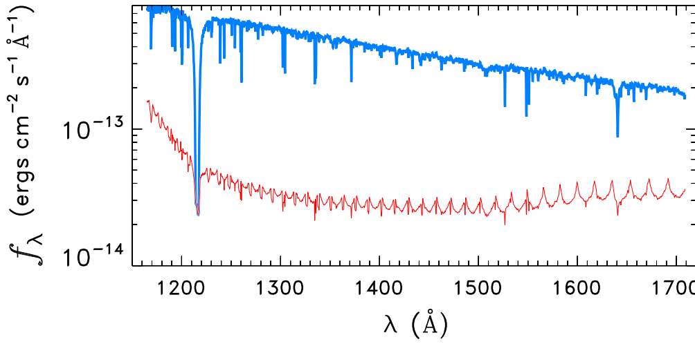
WD0505+012
