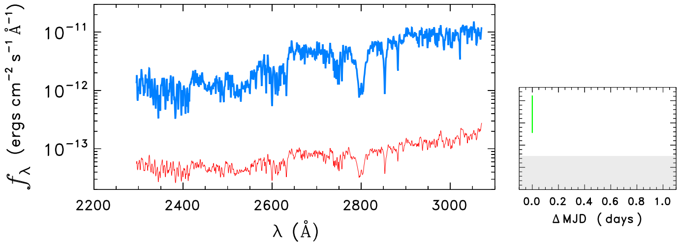
HD187691
