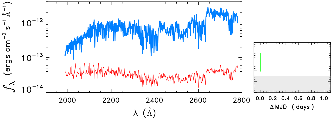
HD190009
