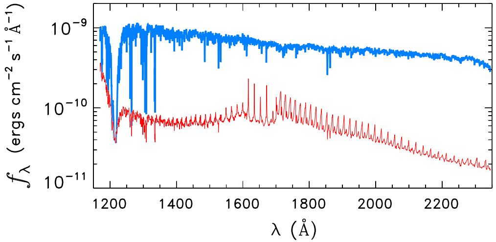
HD147394
