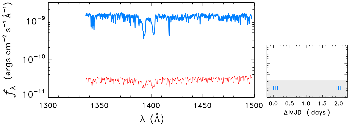
HD24398
