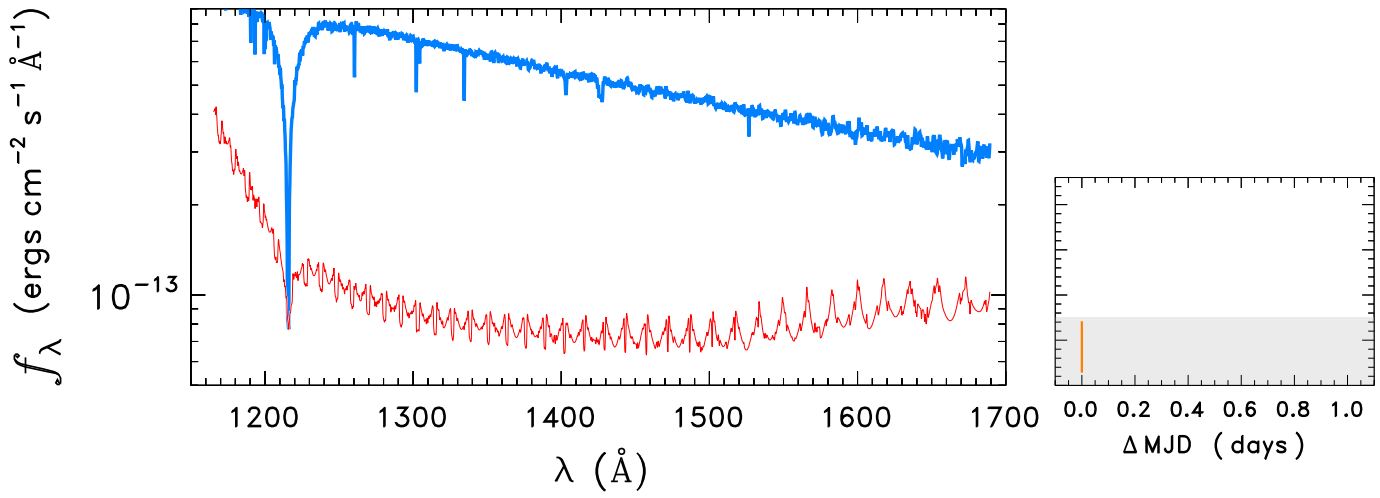
WD2152-548
