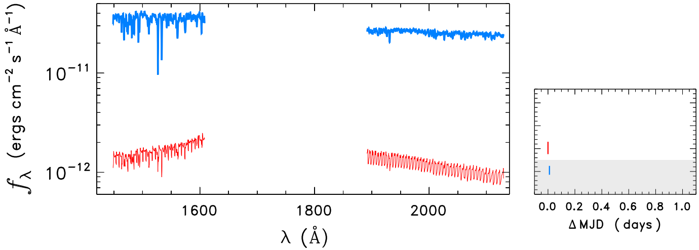
HD109573
