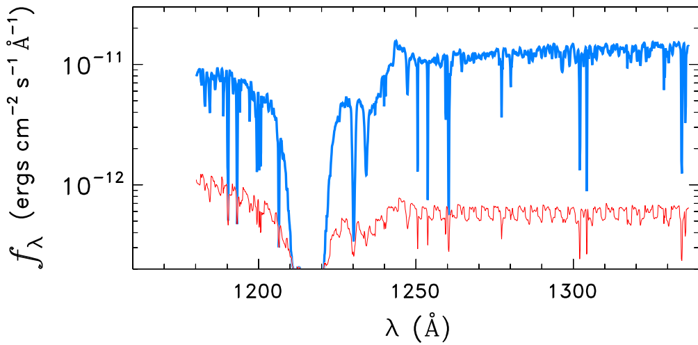
HD115455
