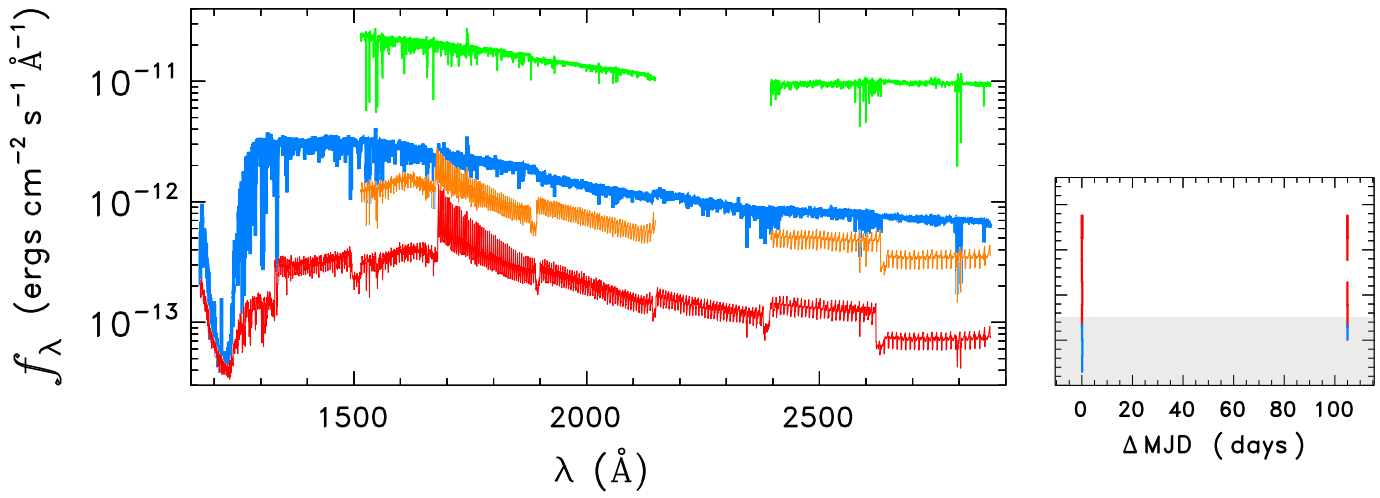
HD100546
