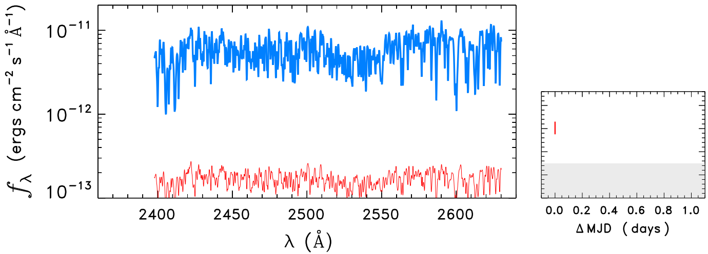
HD109799
