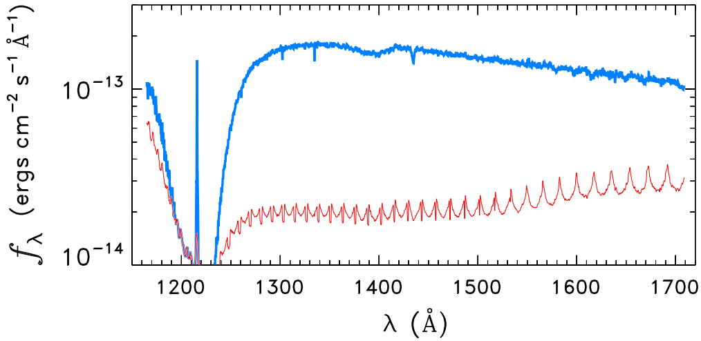
WD0429+176
