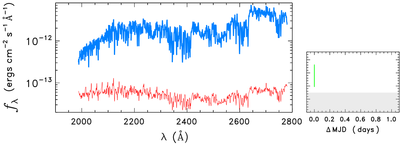
HD184985
