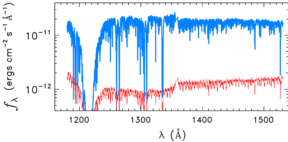
HD106943
