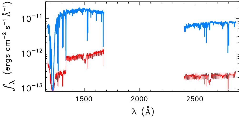
HD102065
