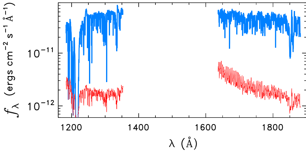
HD106343
