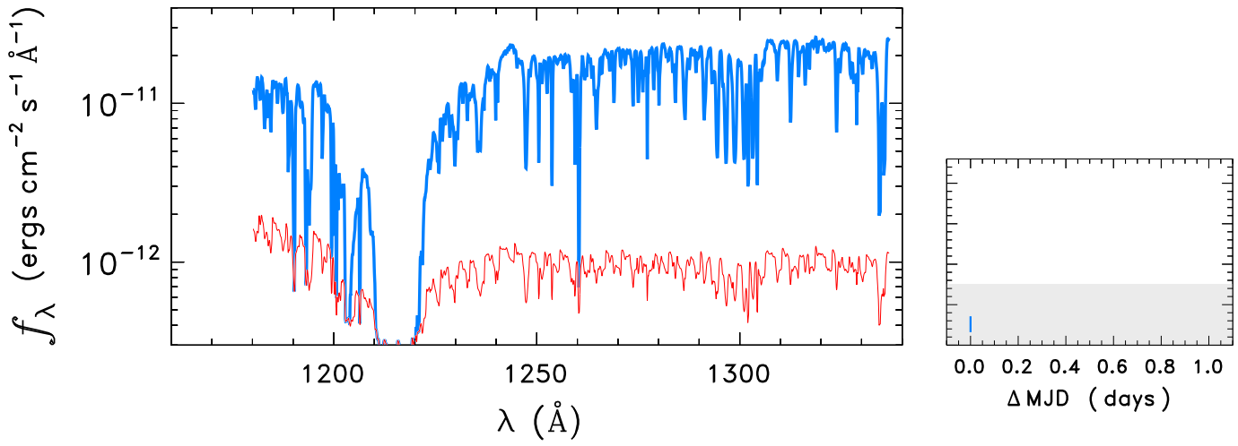
HD111934
