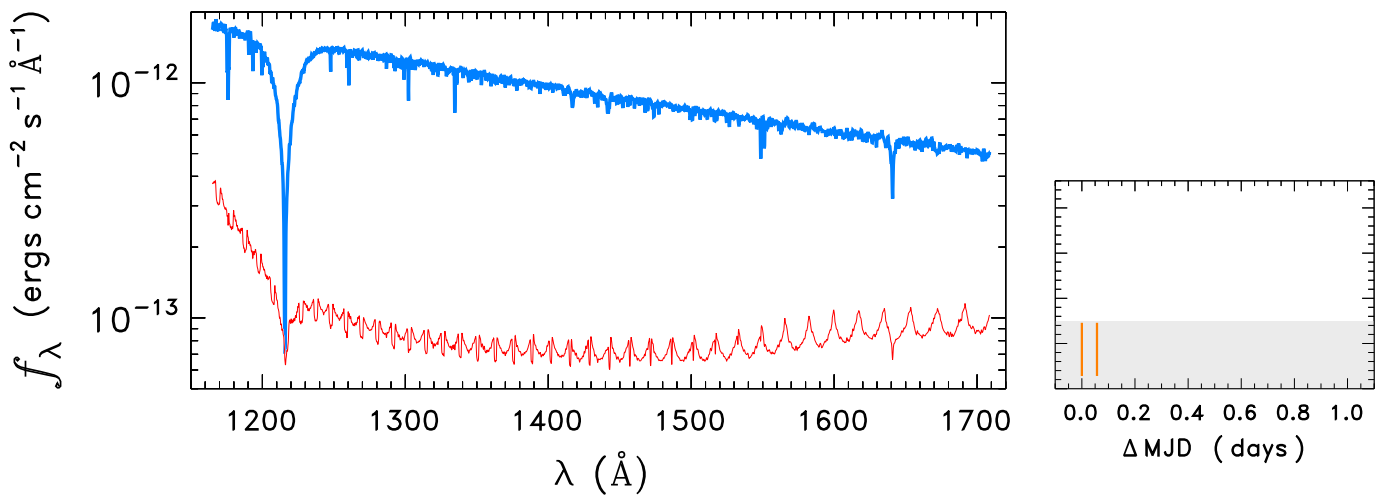
WD0209+085
