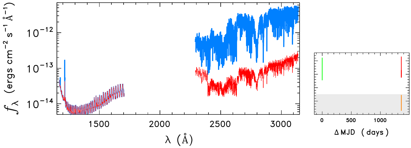
HD184499
