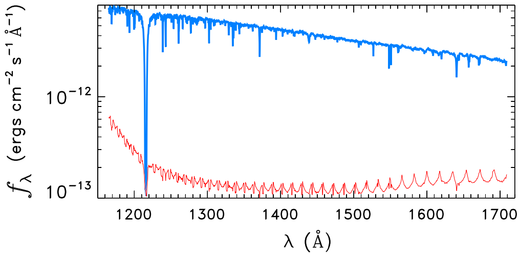
WD0439+466
