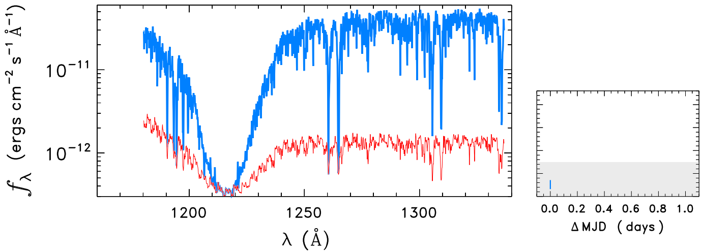
HD1909
