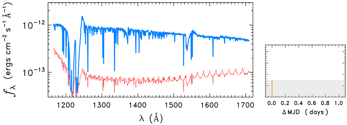
STAR0059-7210a
