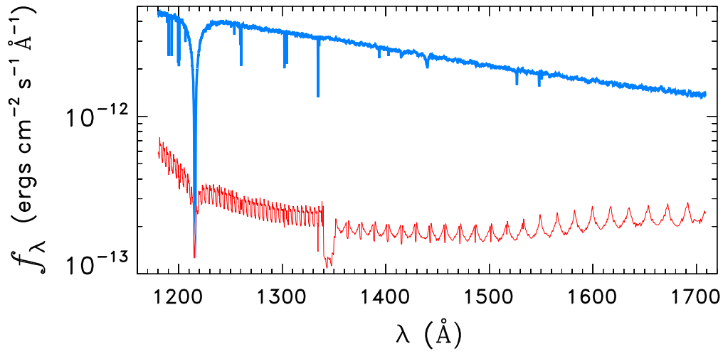
WD2309+105
