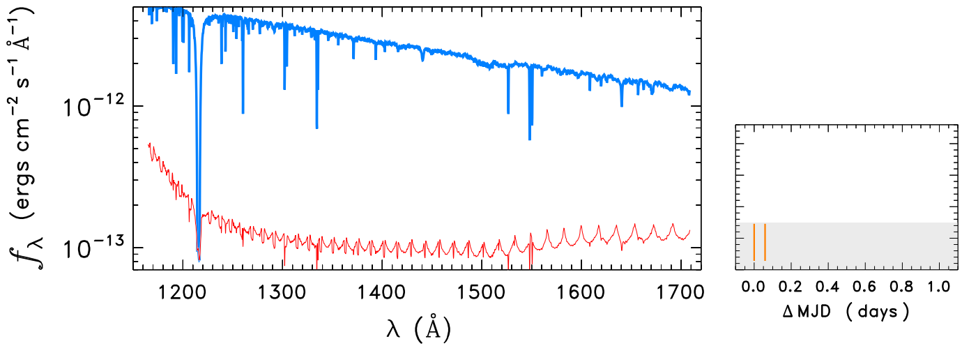
WD2226-210
