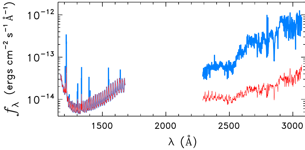
HD116956
