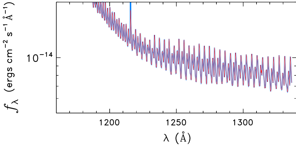
WD0501-289
