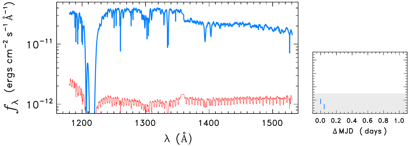
HD24190
