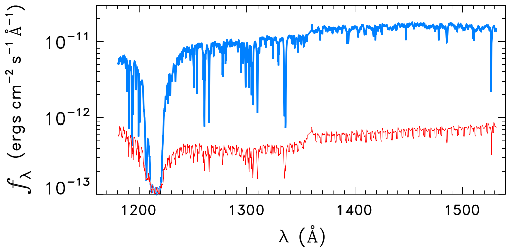
HD147683
