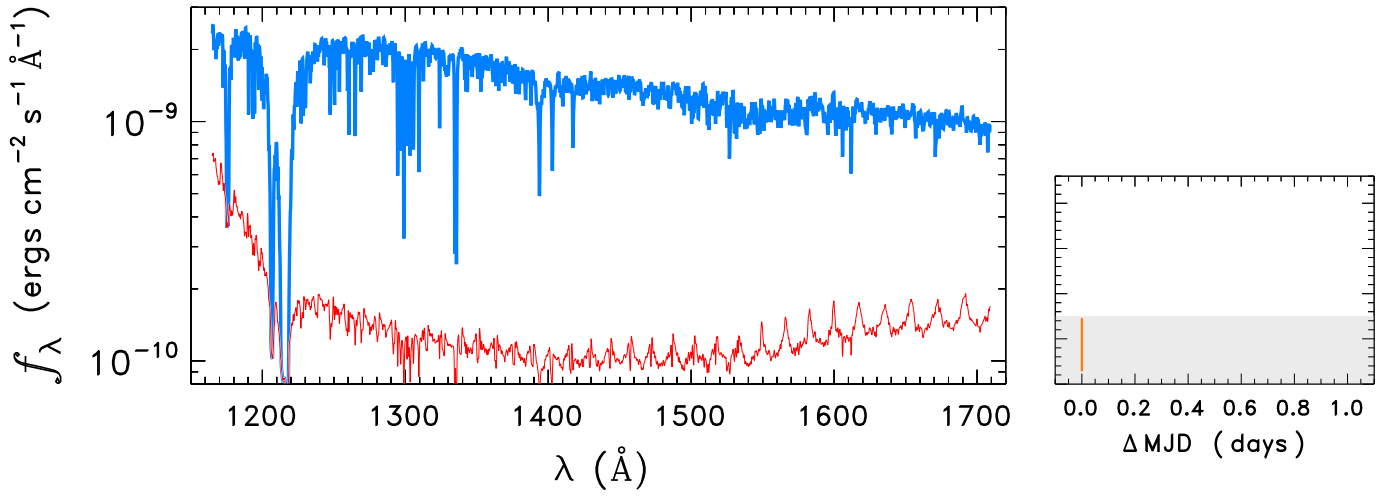
HD112092
