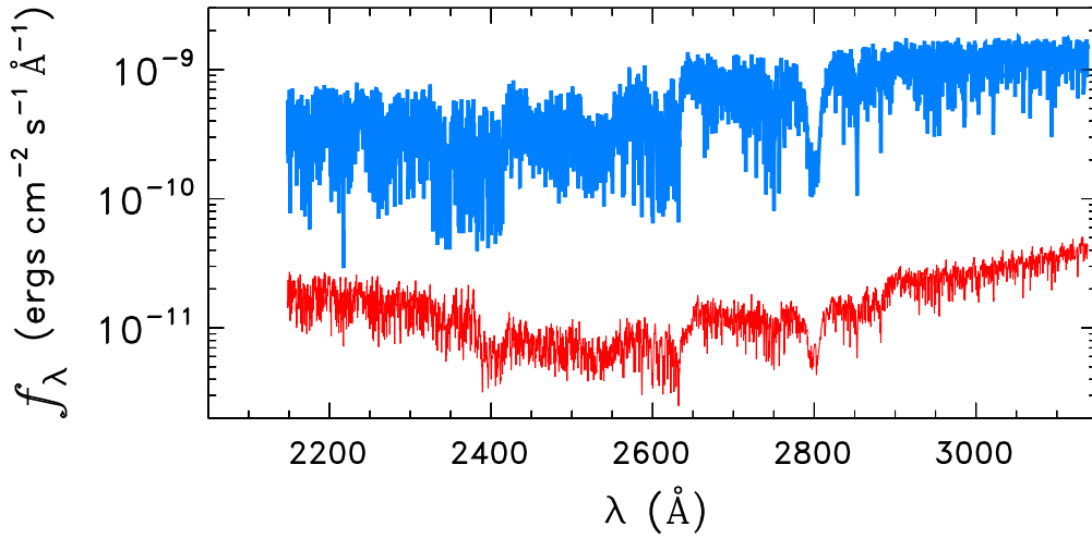
HD61421
