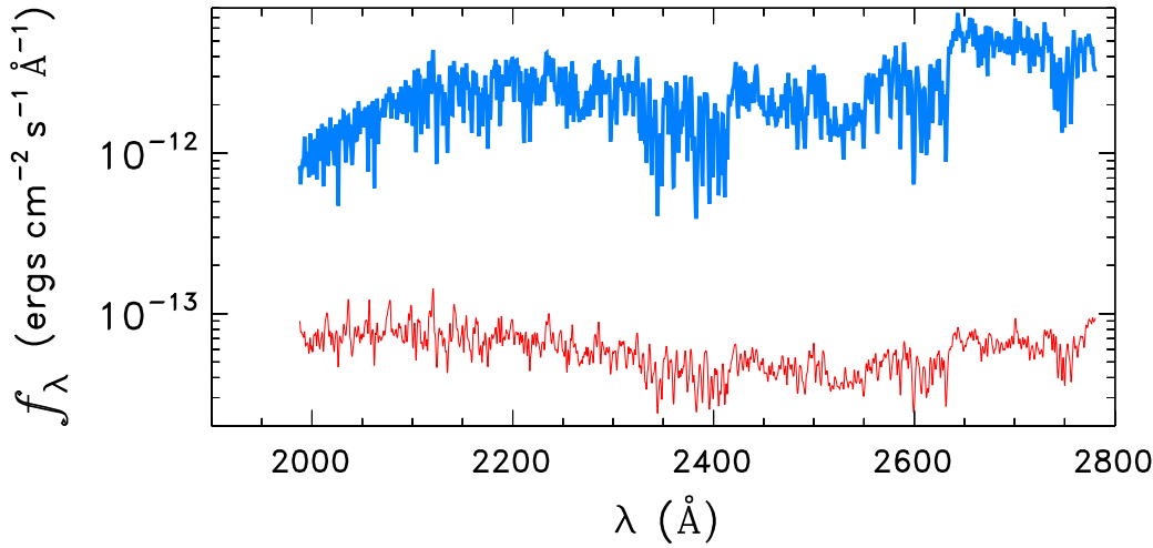
HD191195
