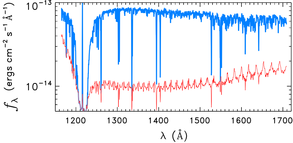
STAR0058-7210a
