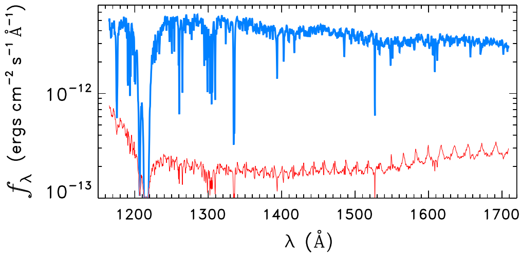
HD187311
