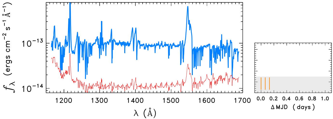
HD108907
