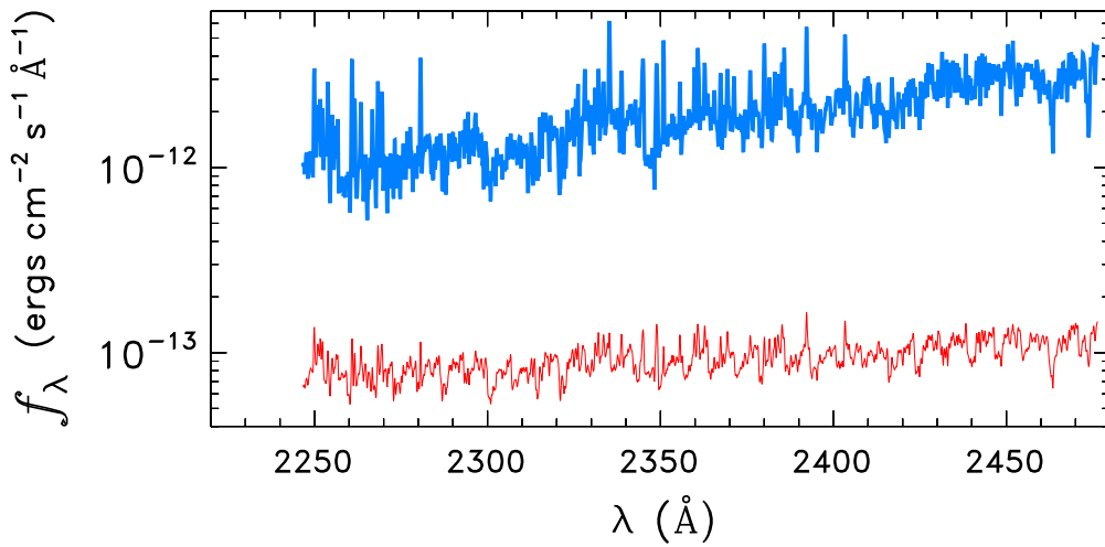
HD62509
