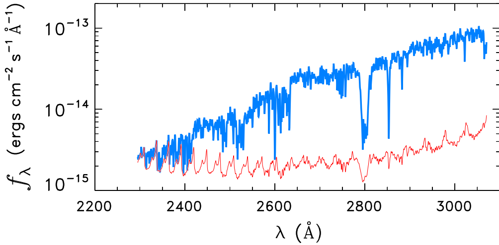
HD186478
