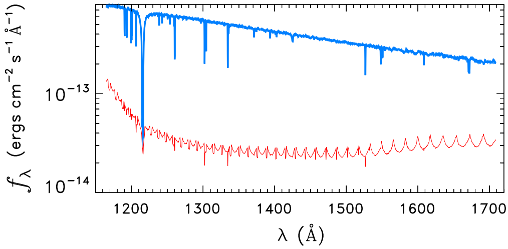
WD0948+534
