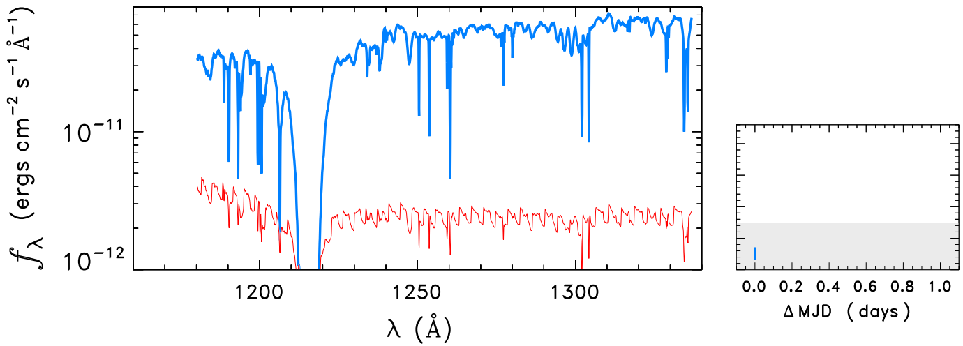
HD198781
