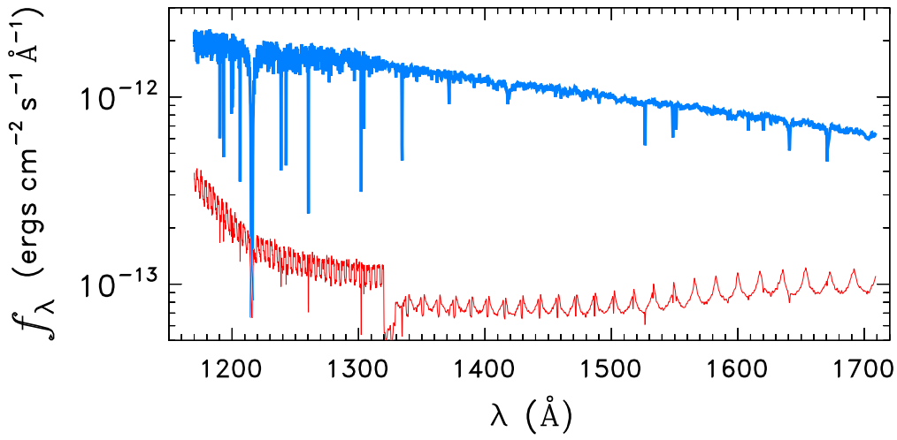
WD1136+667
