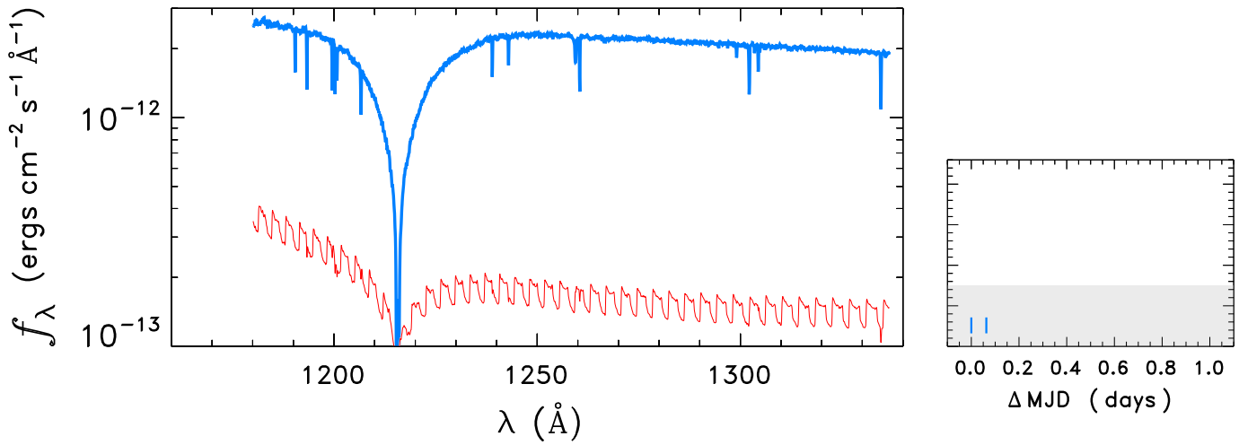
WD0050-332
