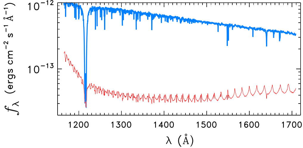
WD2342+806
