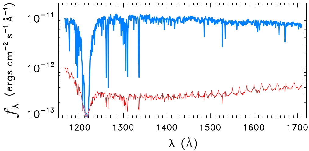
HD191466
