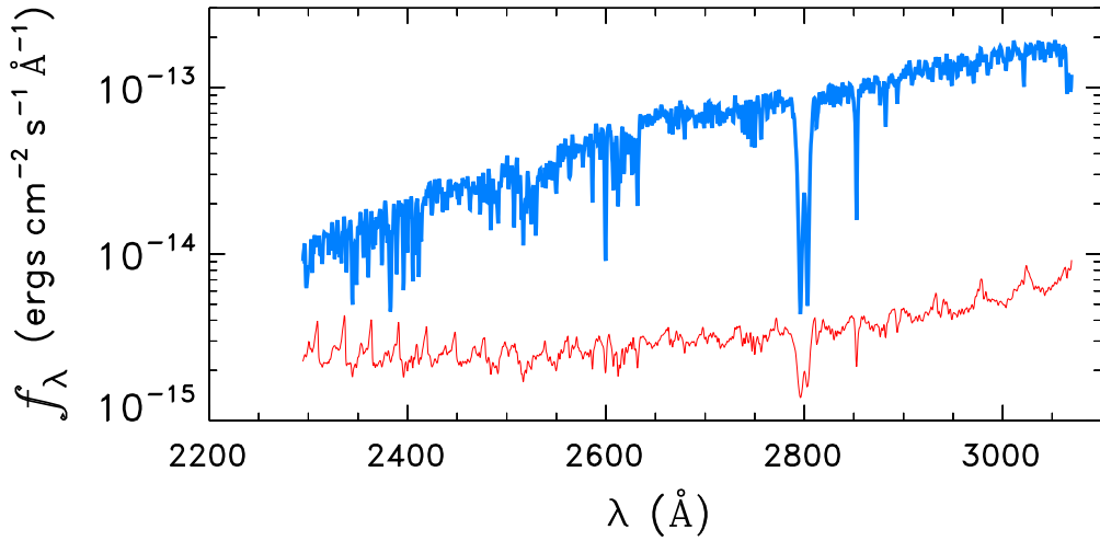
HD115444
