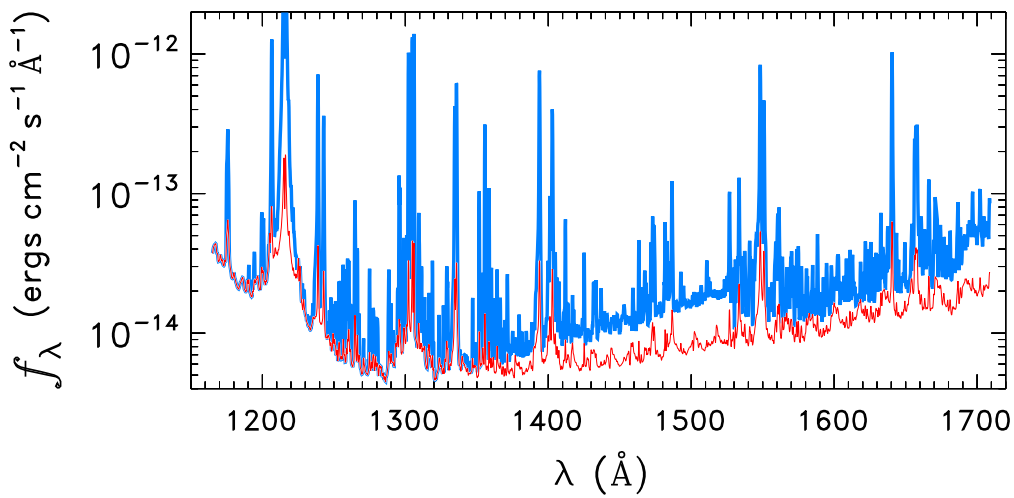
HD93497
