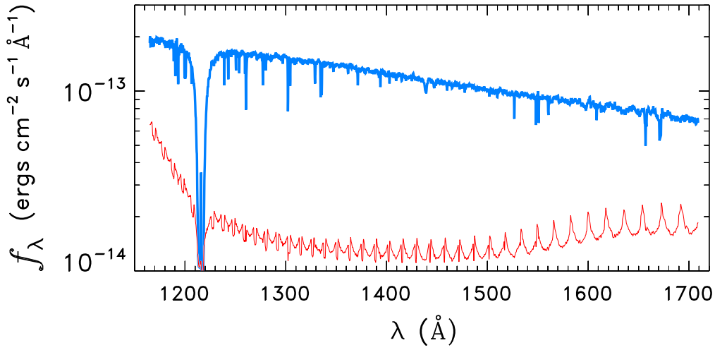
WD0615+655
