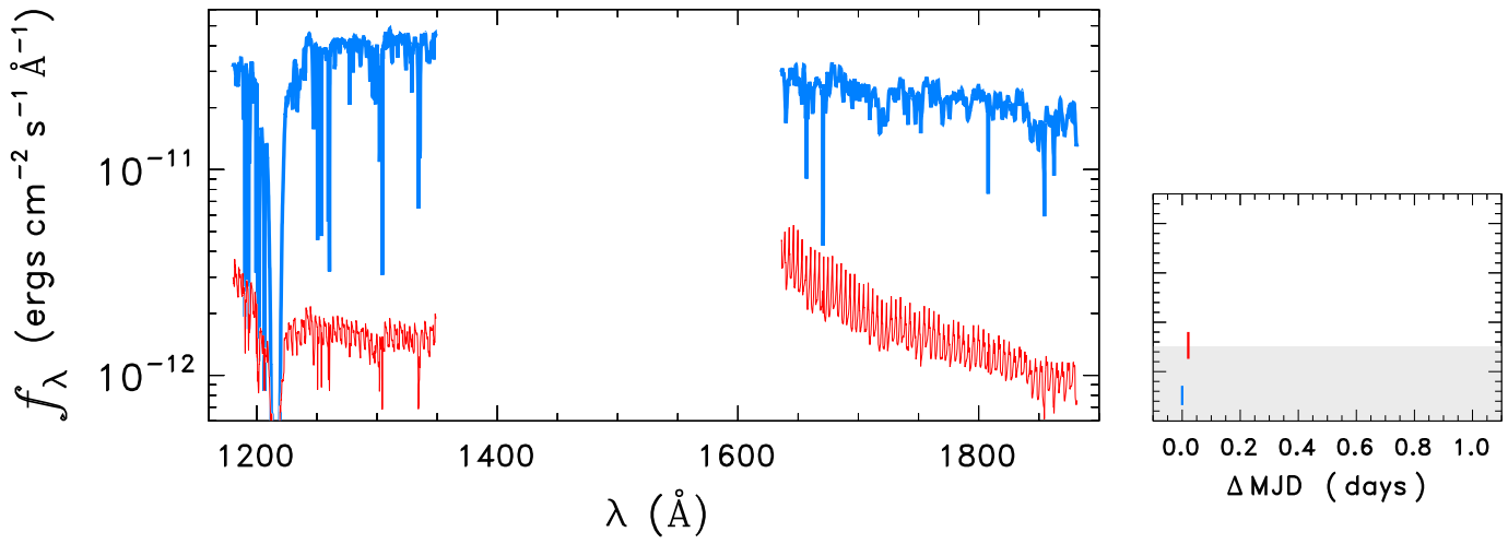
HD109399
