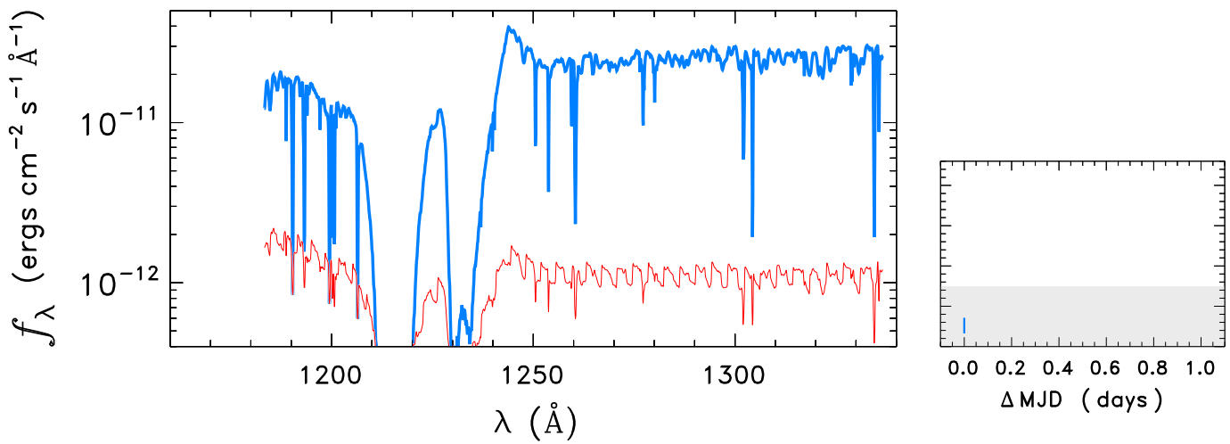
HD157857
