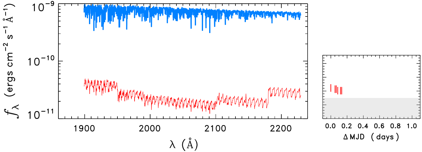
HD16582
