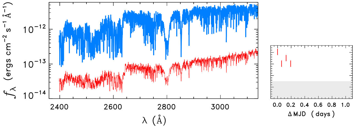
HD157466
