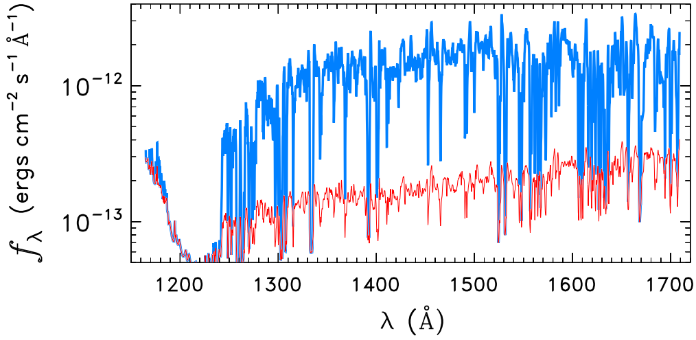
HD93308/POS-ECH1
