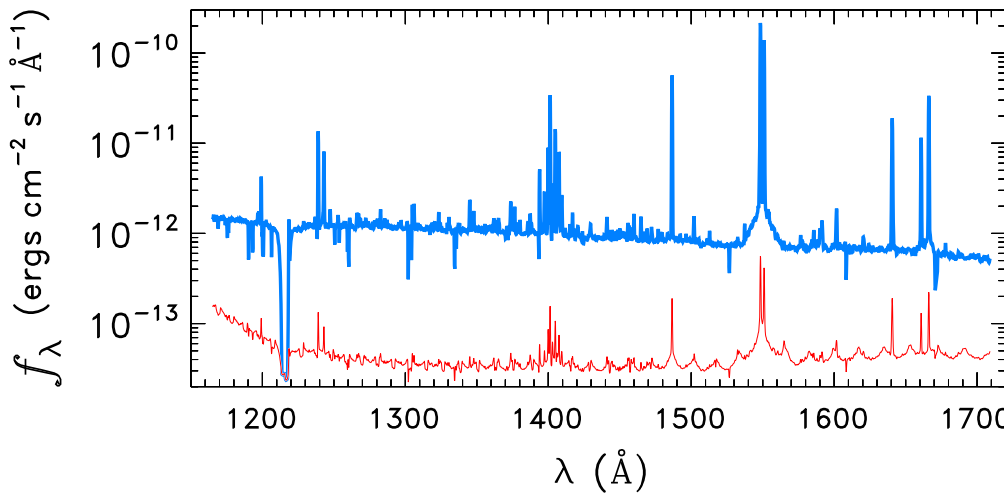
HD117970
