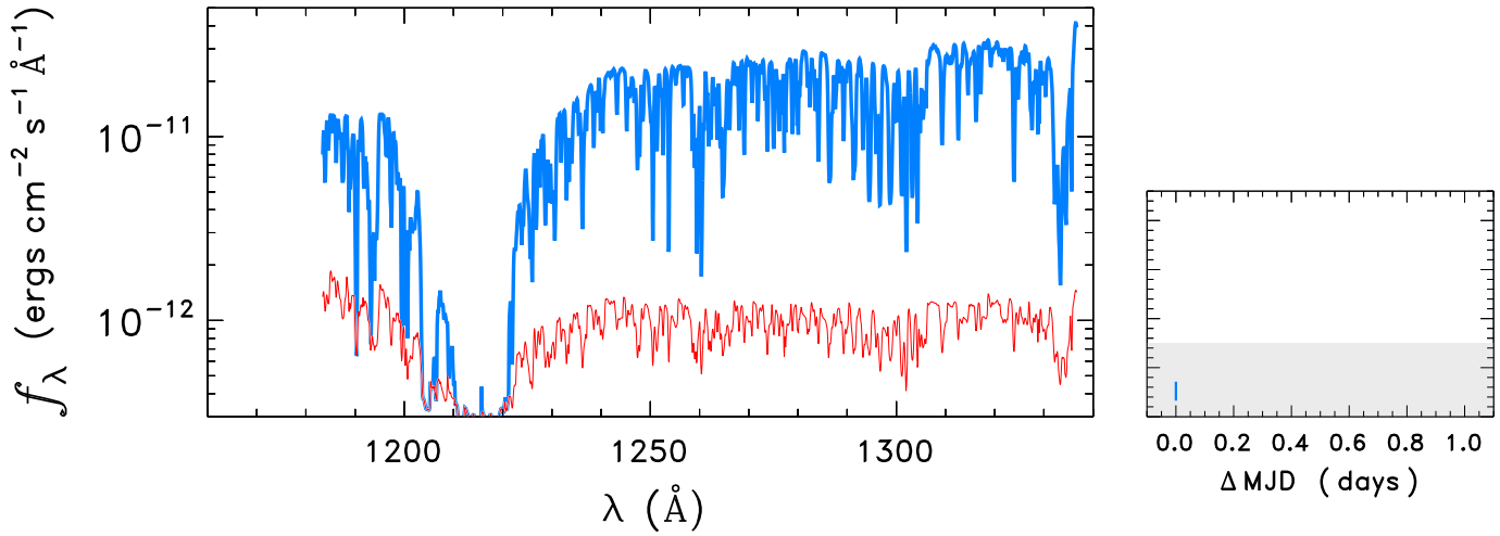
HD198478
