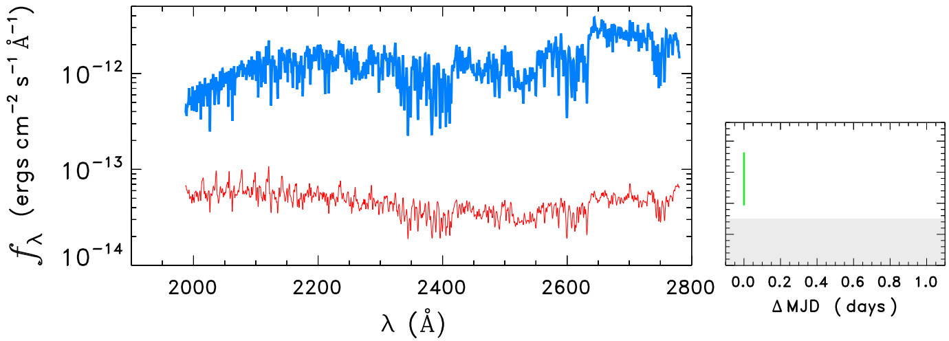
HD157856
