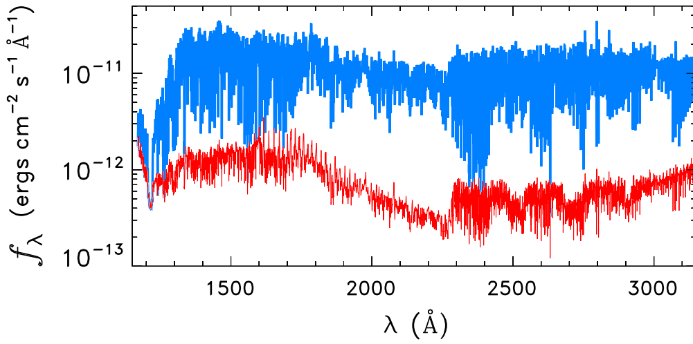
HD60414
