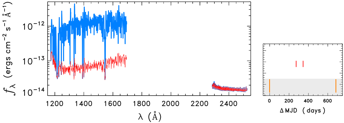
HD184738
