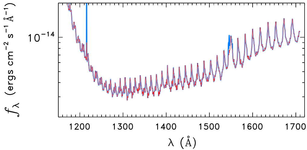
WX-CET
