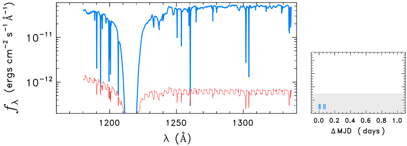
HD165246
