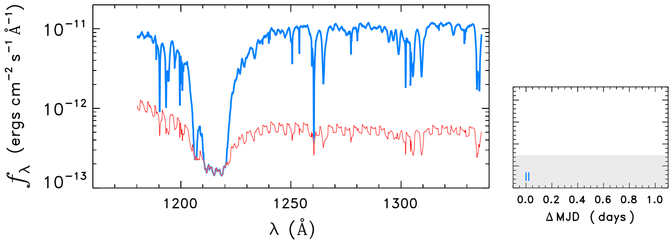
HD112999
