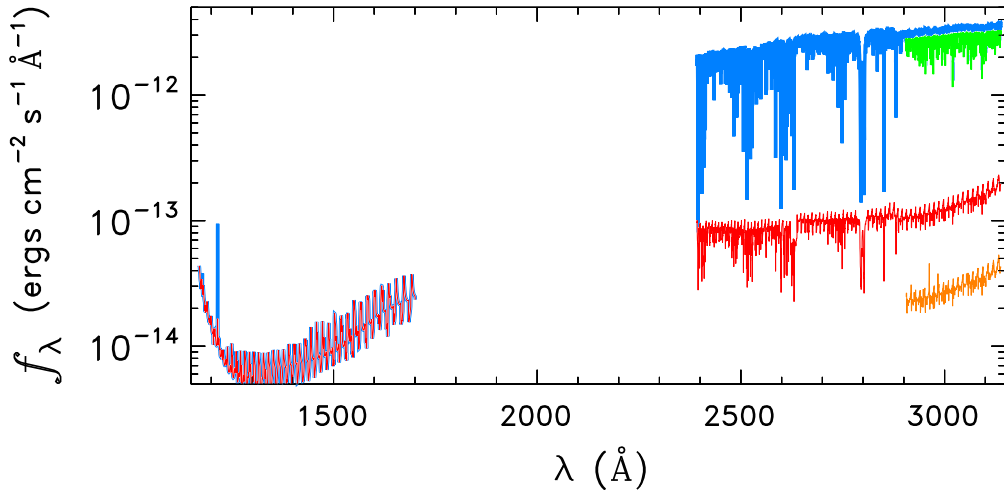
HD140283
