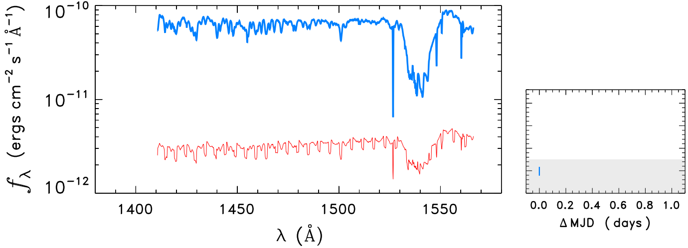
HD101131
