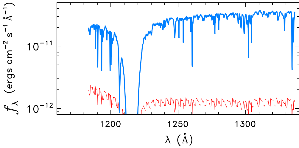
HD185418
