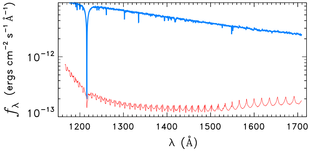
WD0232+035
