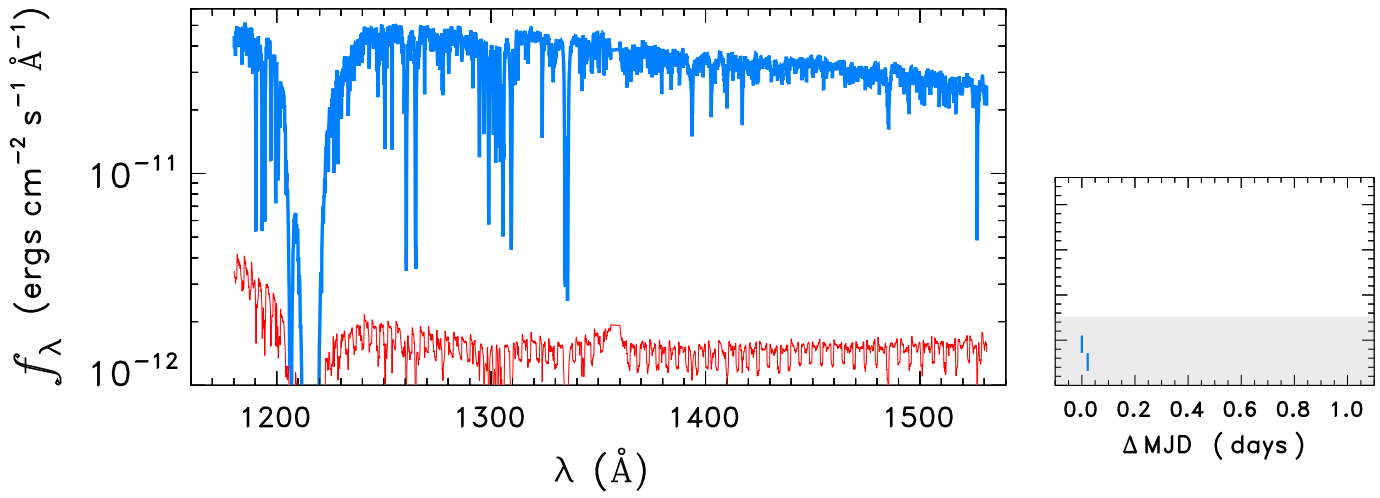
HD108610
