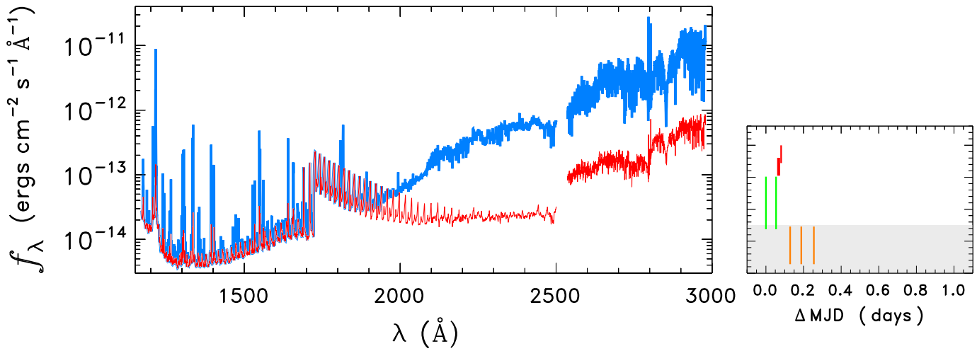
HD165341
