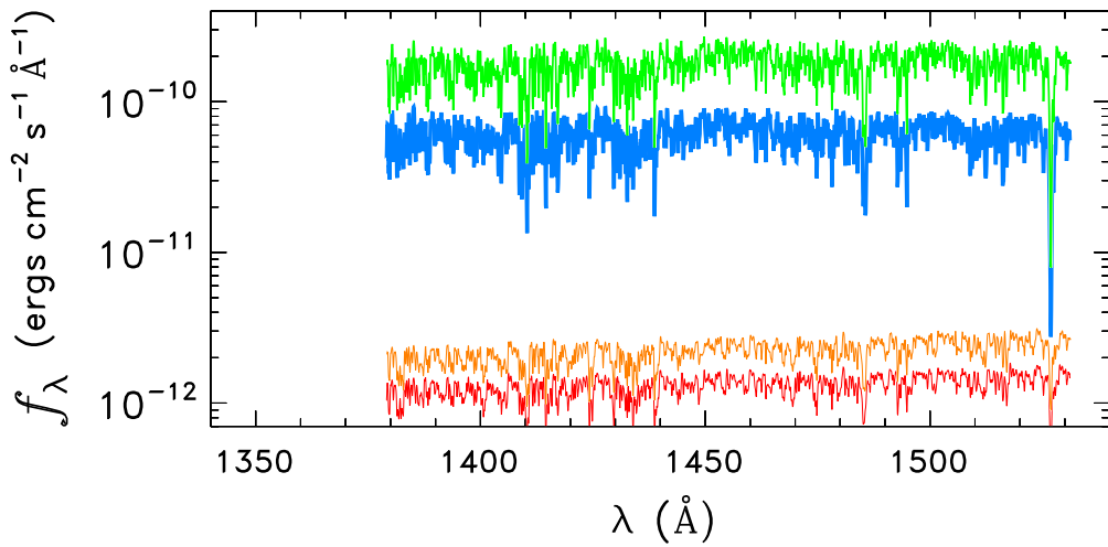
HD141556
