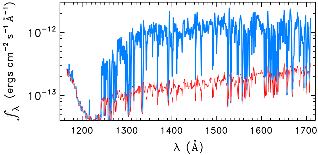
HD93308/POS-ECH2
