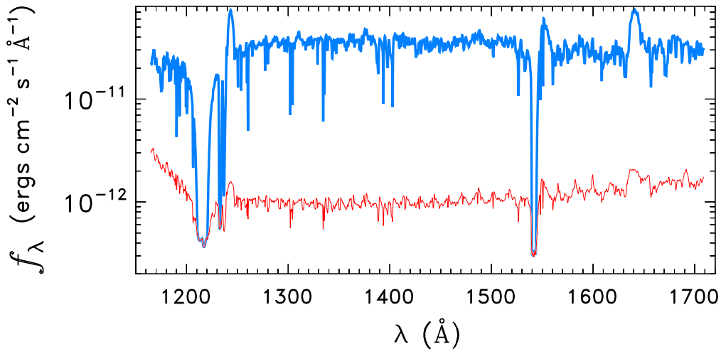
HD190918
