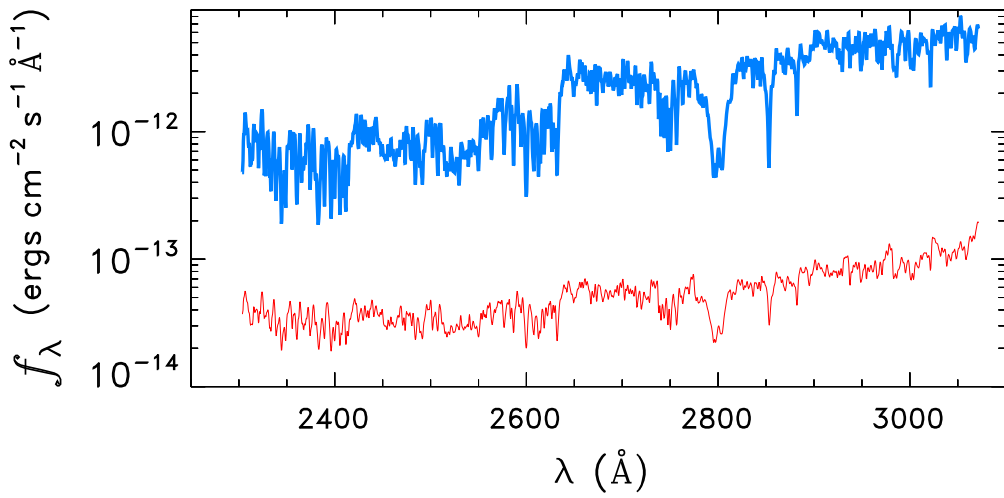
HD102634
