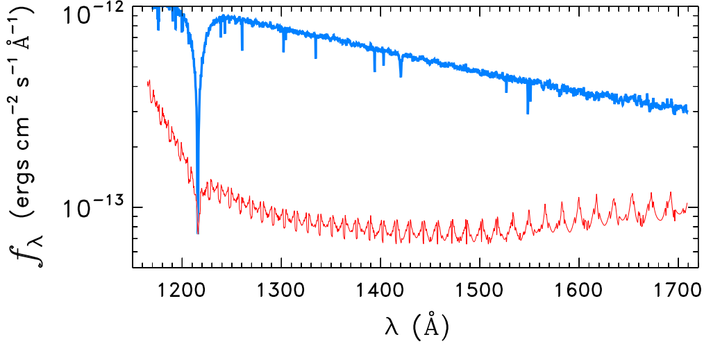
WD1029+537
