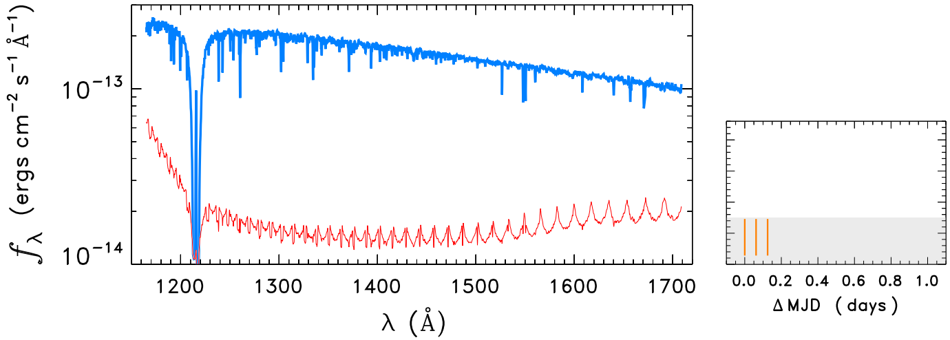
WD2218+706
