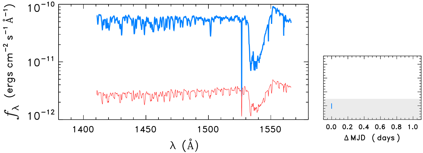
HD101190
